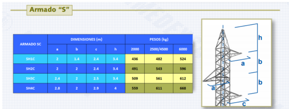
Figura 3. Detalla constructivo apoyo de celosía con armado tipo "S"
